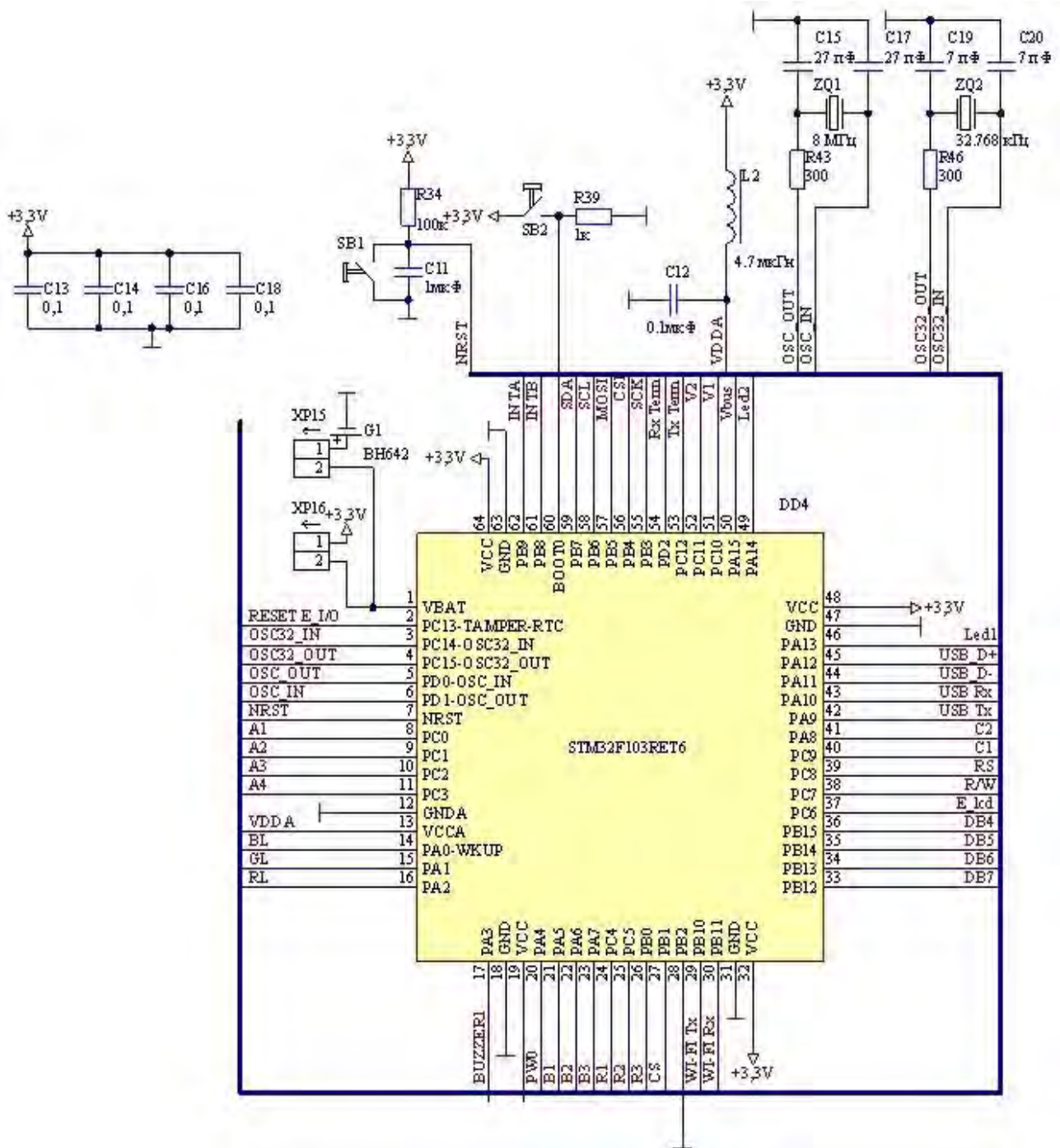
Рисунок 1 – Схема контроллера STM32
